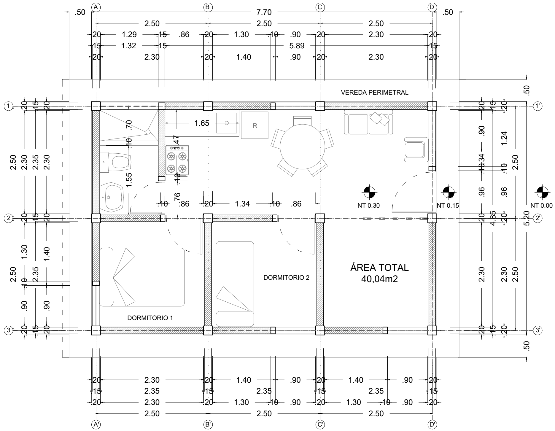
PLANTA ARQUITECTÓNICA
